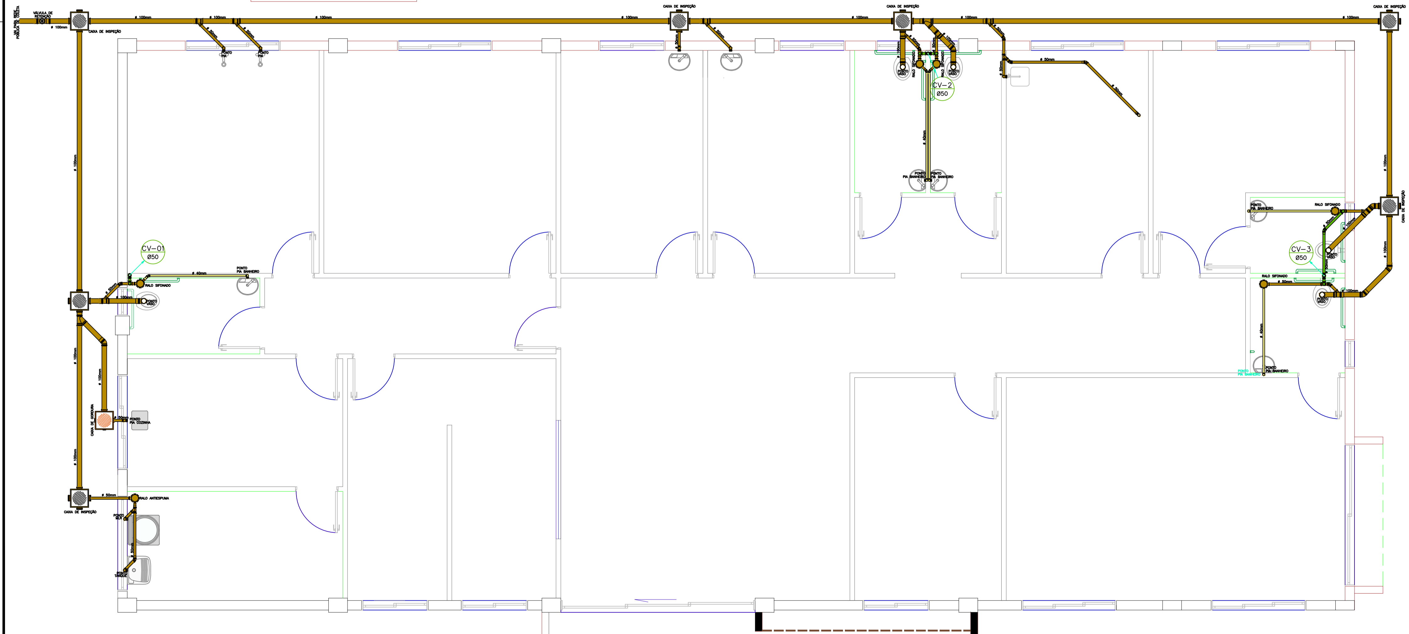
PLANTA BAIXA - SANITÁRIO ESCALA : 1/50
