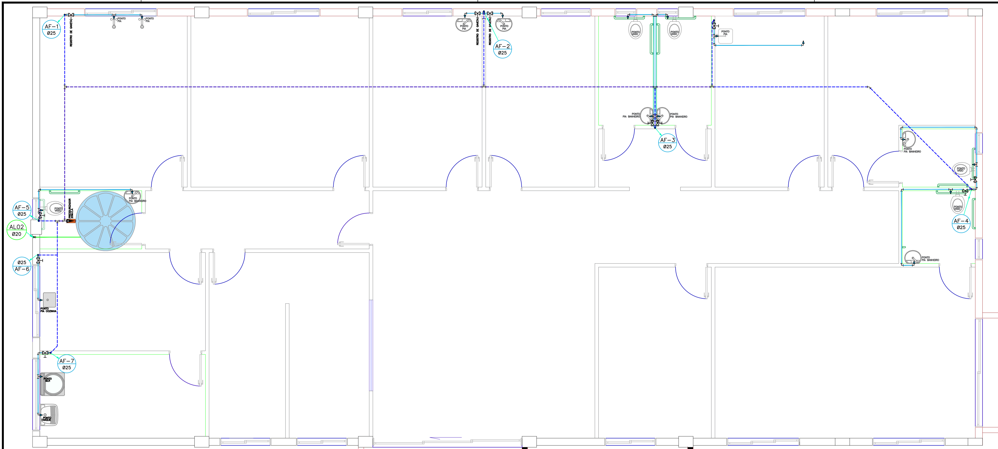
PLANTA BAIXA - HIDRÁULICA ESCALA : 1/50
