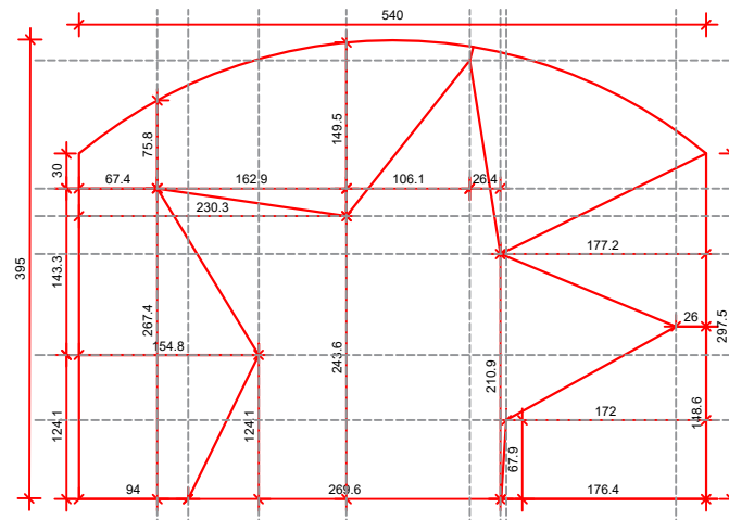
ESTRUTURA - PORTAIS PRAÇA LAURO MULLER ESC.: 1: 50
