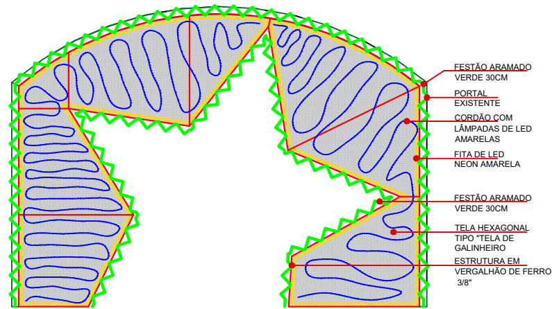
VISTA FRONTAL - PORTAIS PRAÇA LAURO MULLER ESC.: 1: 50
