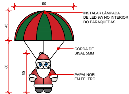
VISTA FRONTAL ESC.: 1: 25
