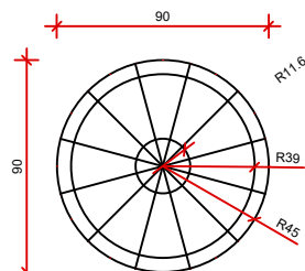
VISTA SUPERIOR ESC.: 1: 25
