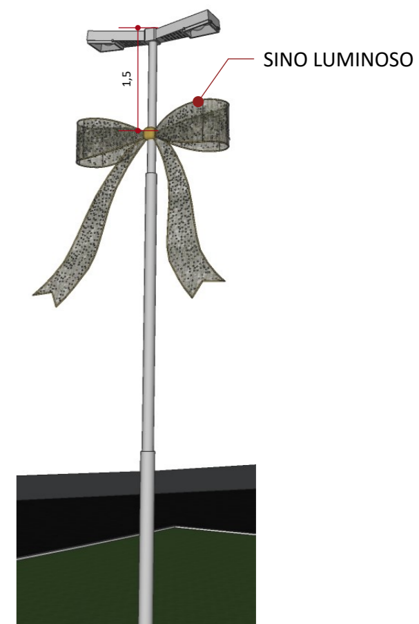
3 PERSPECTIVA DOS POSTES 01 SEM ESCALA
