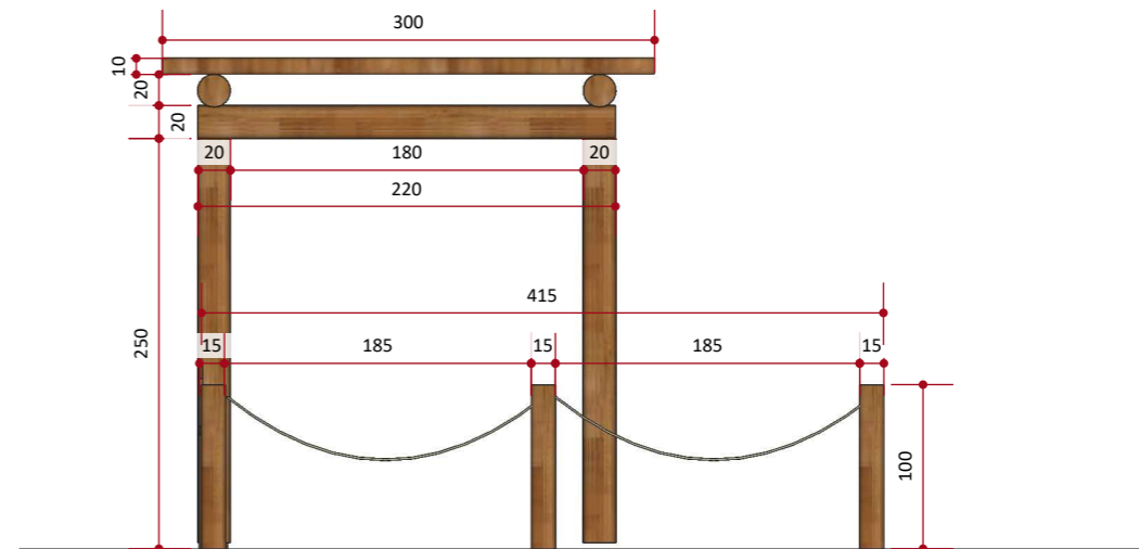
2 VISTA LATERAL PRESÉPIO 01 ESC. 1/50
