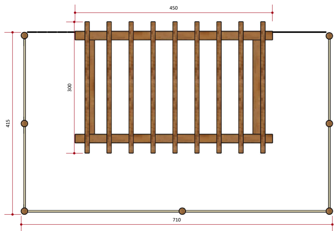
3 VISTA SUPERIOR PRESÉPIO 01 ESC. 1/50
