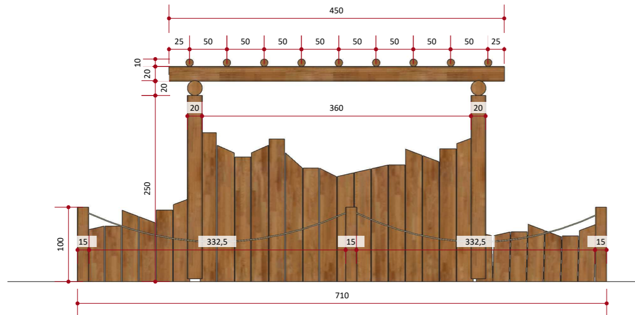
1 VISTA FRONTAL PRESÉPIO 01 ESC. 1/50
