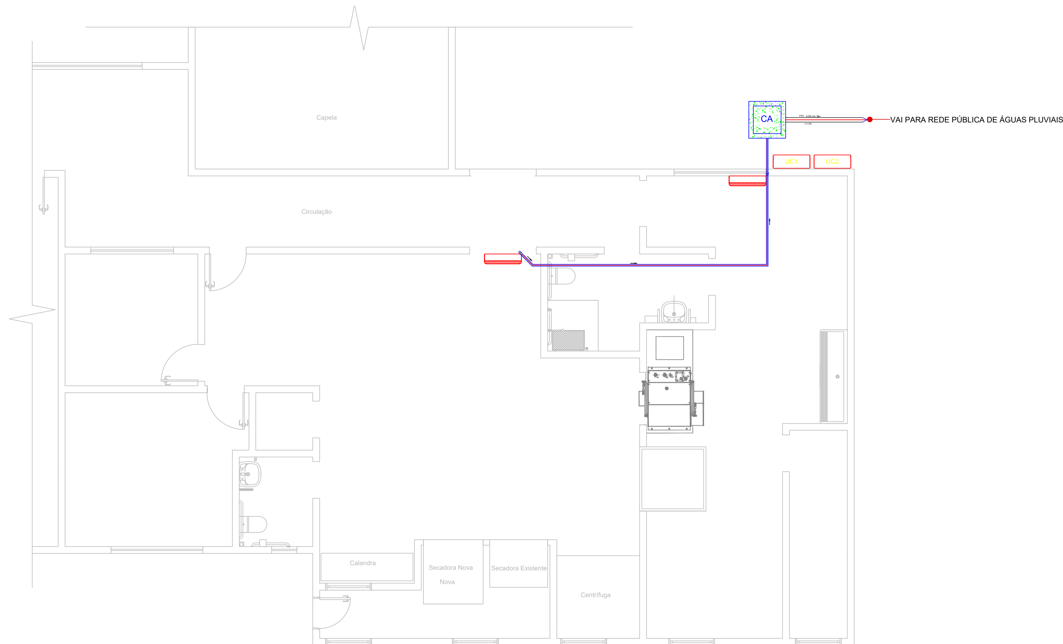
PLANTA BAIXA - CLIMATIZAÇÃO ESC.: 1:50
