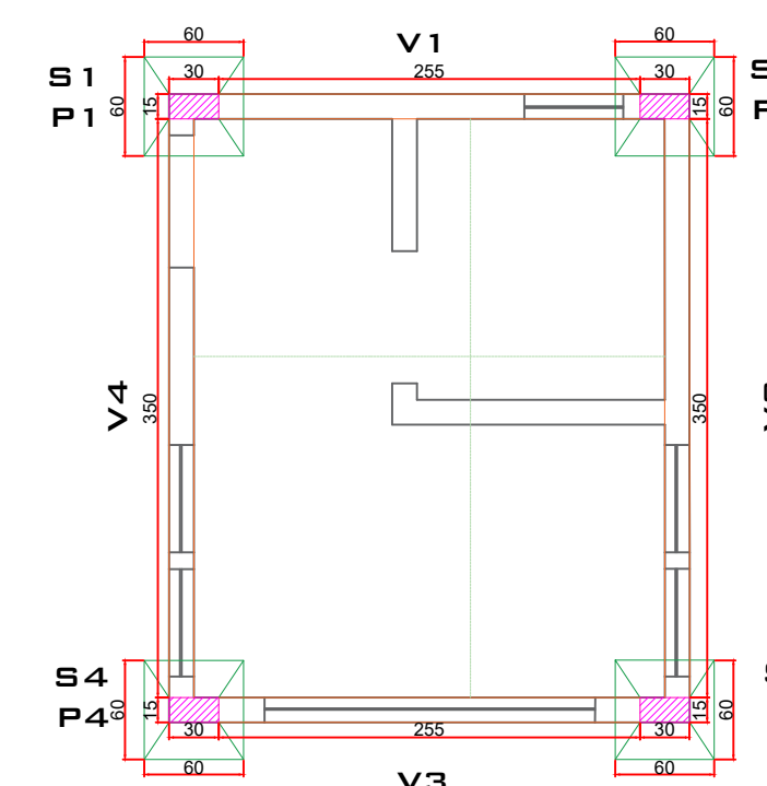
SAPATAS E BALDRAMES esc.:...:1:50
