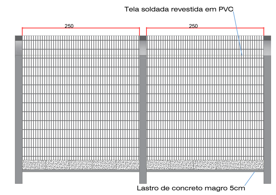
DETALHES DO ALAMBRADO 02 esc.:...:1:50
