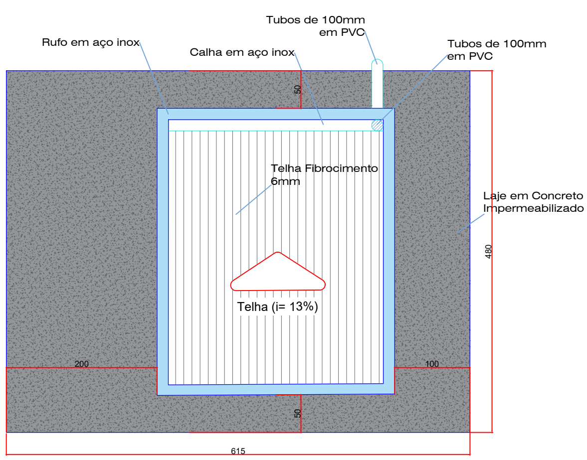
COBERTURA esc.:...:1:50
