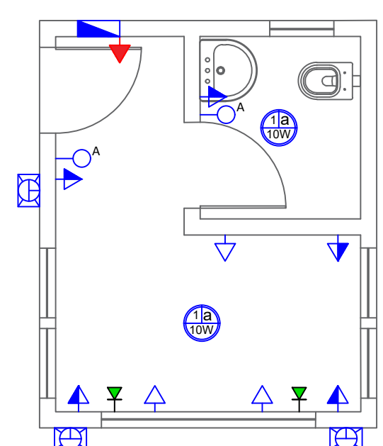
PONTOS ELÉTRICOS esc.:...:1:50
