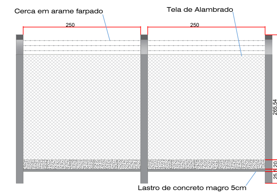
DETALHES DO ALAMBRADO 01 esc.:...:1:50
