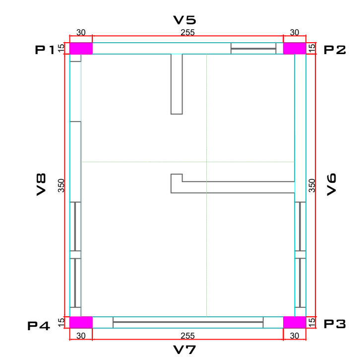
VIGAS SUPERIORES esc.:...:1:50
