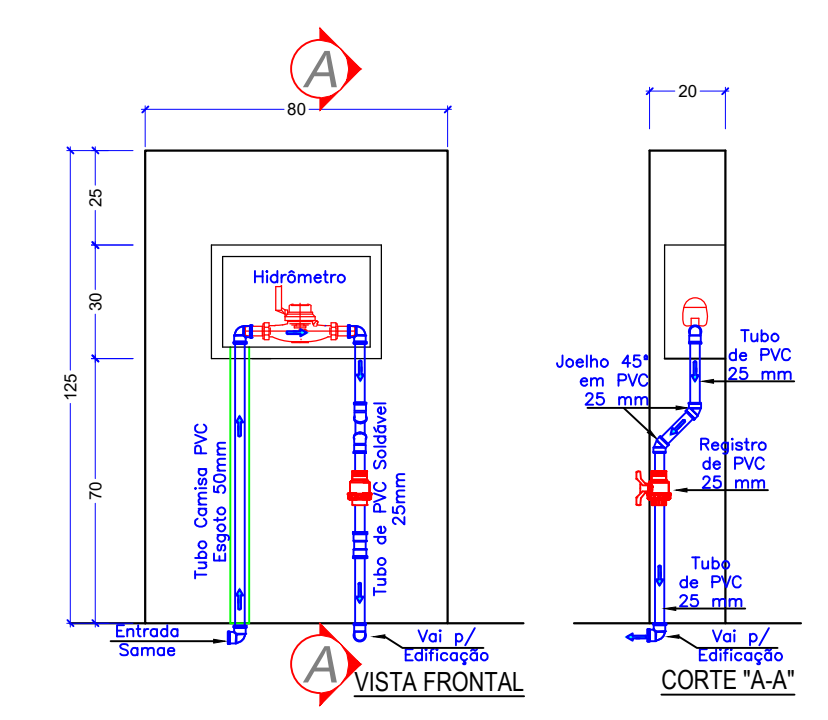
PADRÃO DE ENTRADA SAMAE (Detalhe Genérico) esc.:...:1:20
