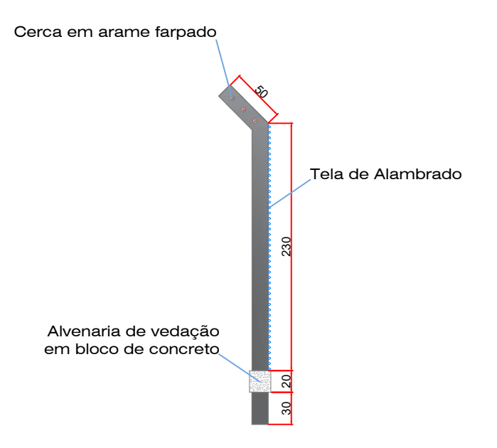
DETALHES DO ALAMBRADO esc.:...:1:50
