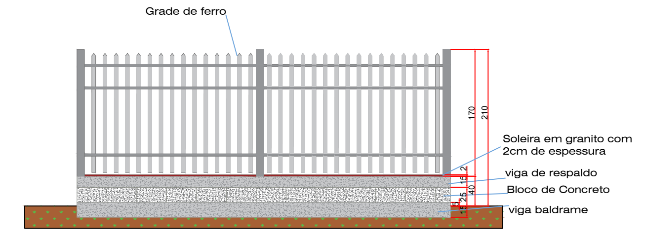
DETALHES DO GRADIL esc.:...:1:50
