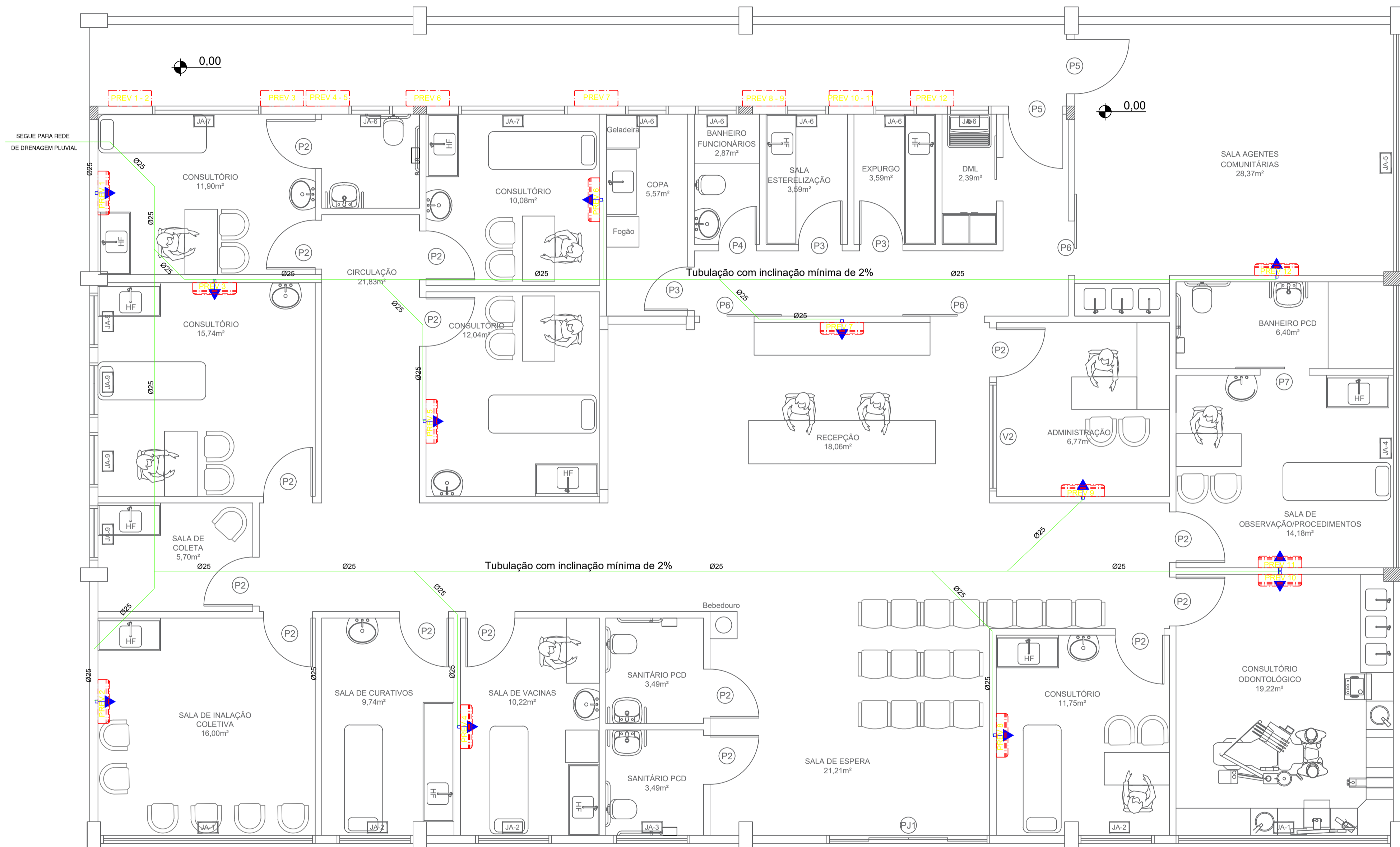
PLANTA BAIXA_ CLIMATIZAÇÃO_ DRENAGEM ESC.: 1: 50
