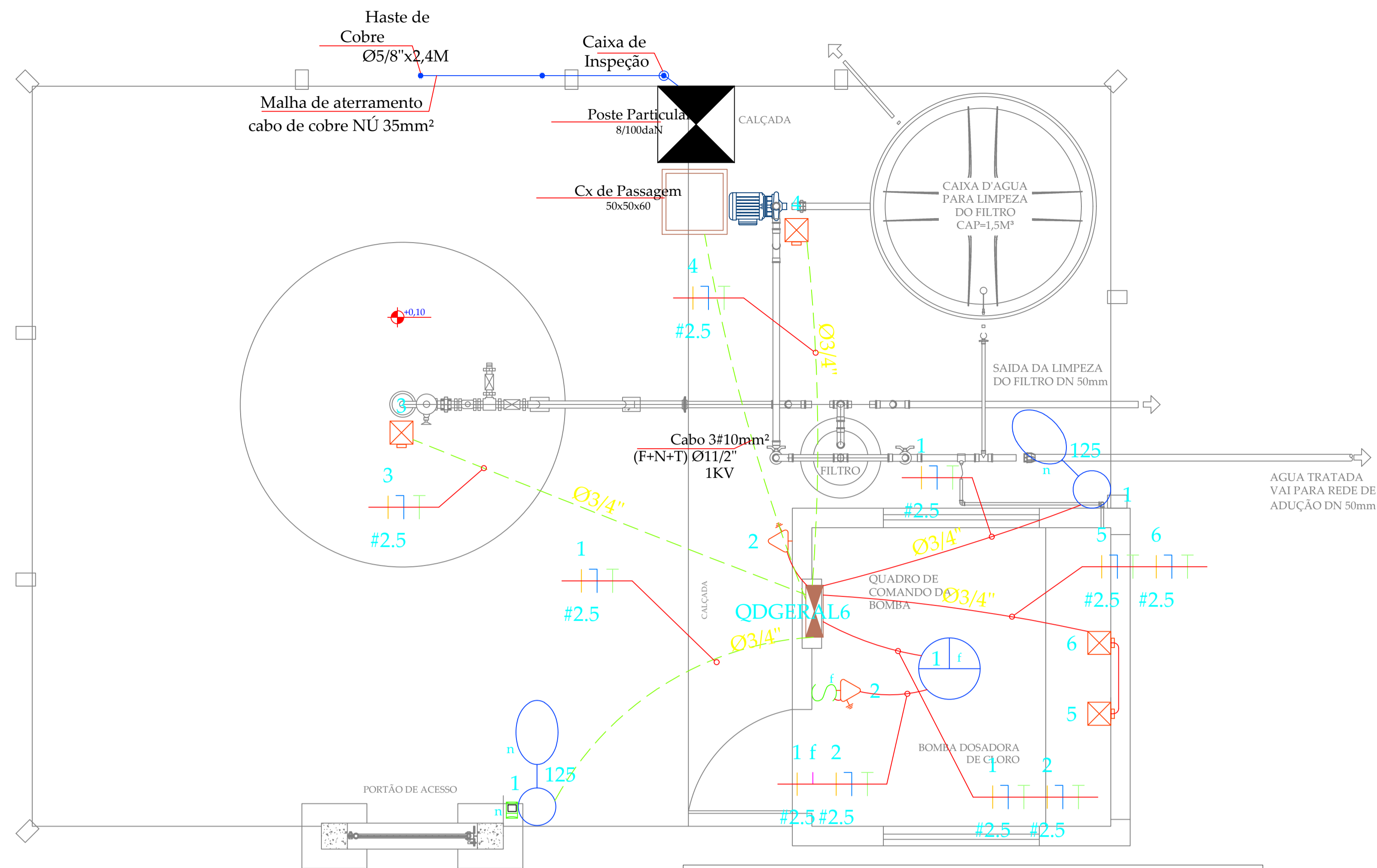
1 PLANTA BAIXA - POÇO 16 ESCALA 1:25
