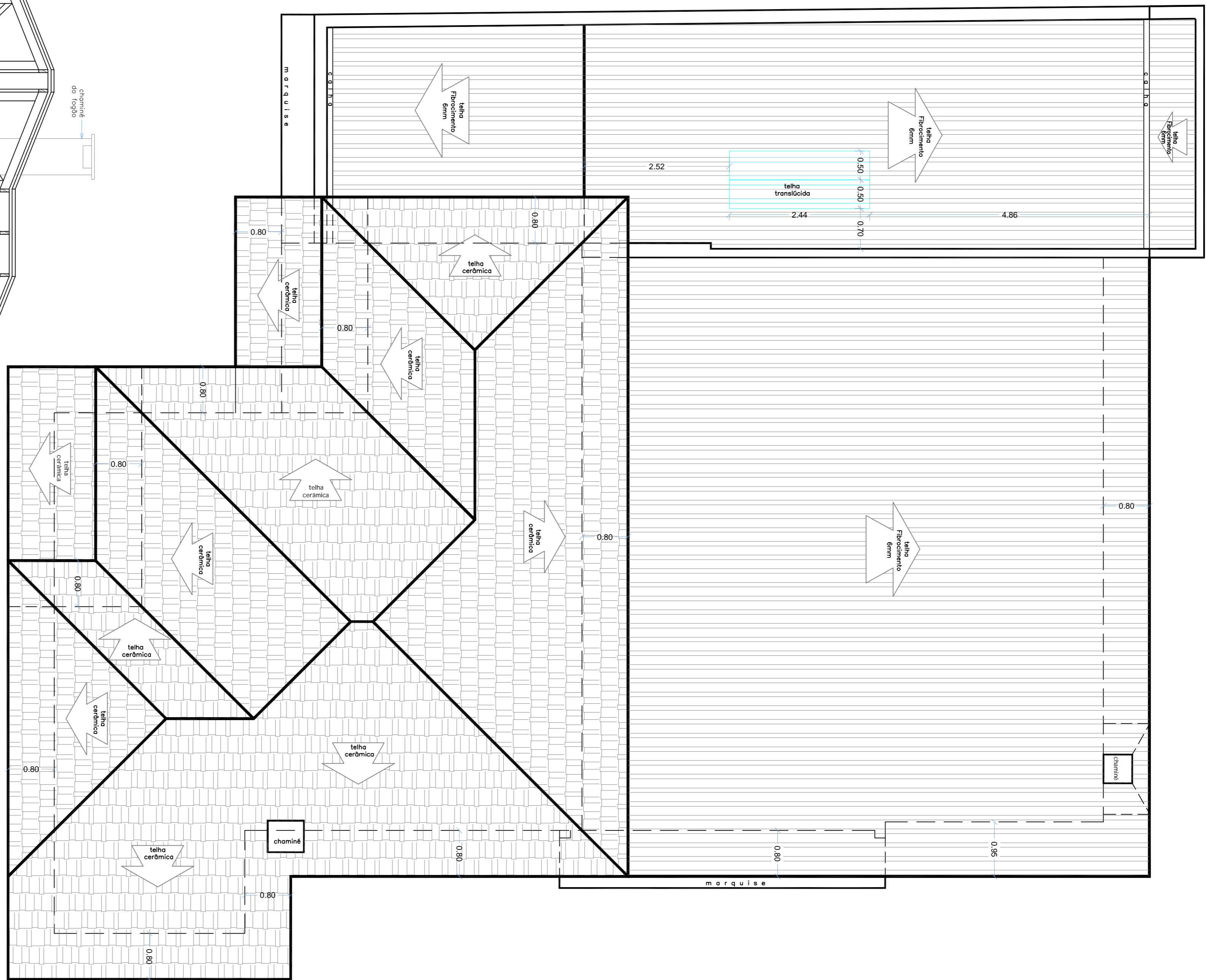
COBERTURA ESCALA..... 1:50
