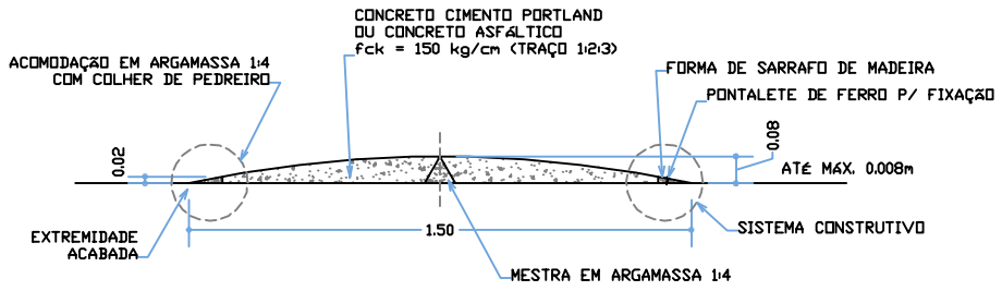
CORTE A-A
