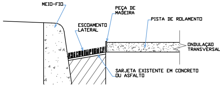
CORTE B-B
