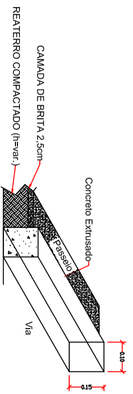
DETALHE - MEIO-FIO S/ ESCALA
