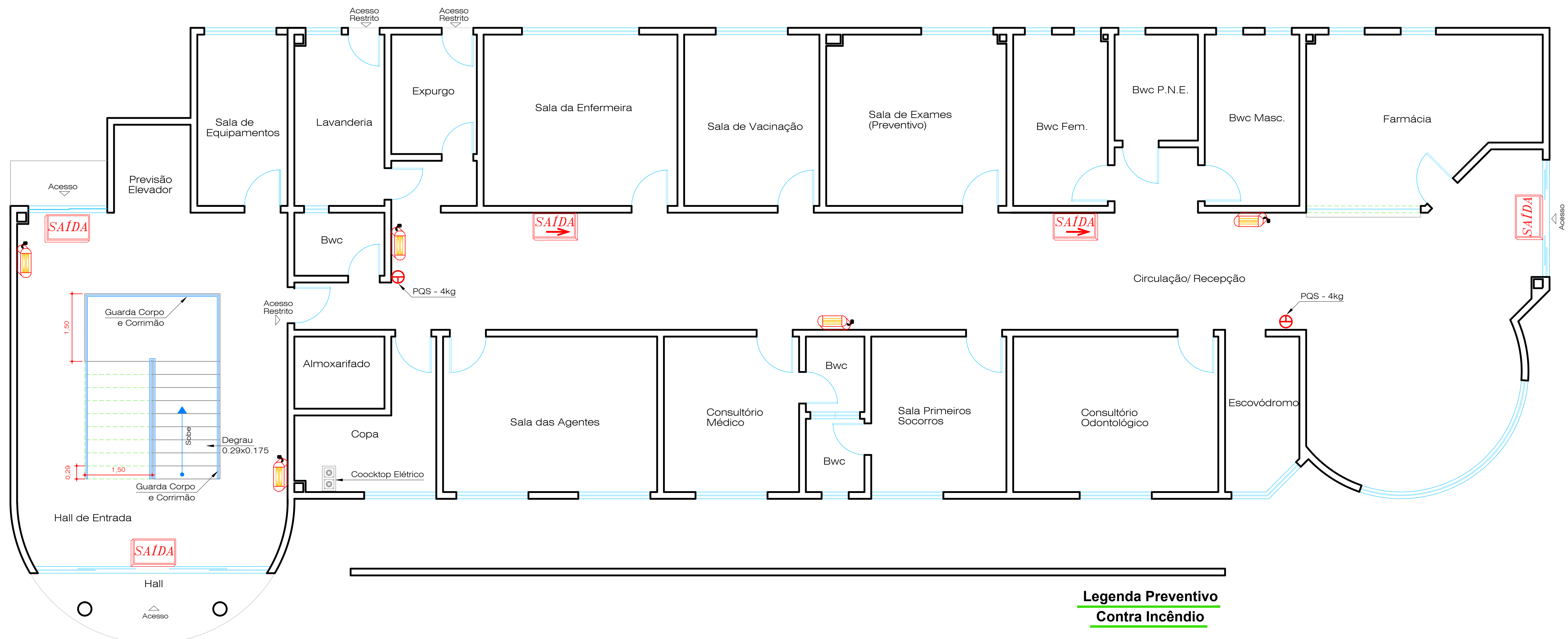
Planta de Preventivo Contra Incêndio - Pav. Térreo Esc. 1:50
