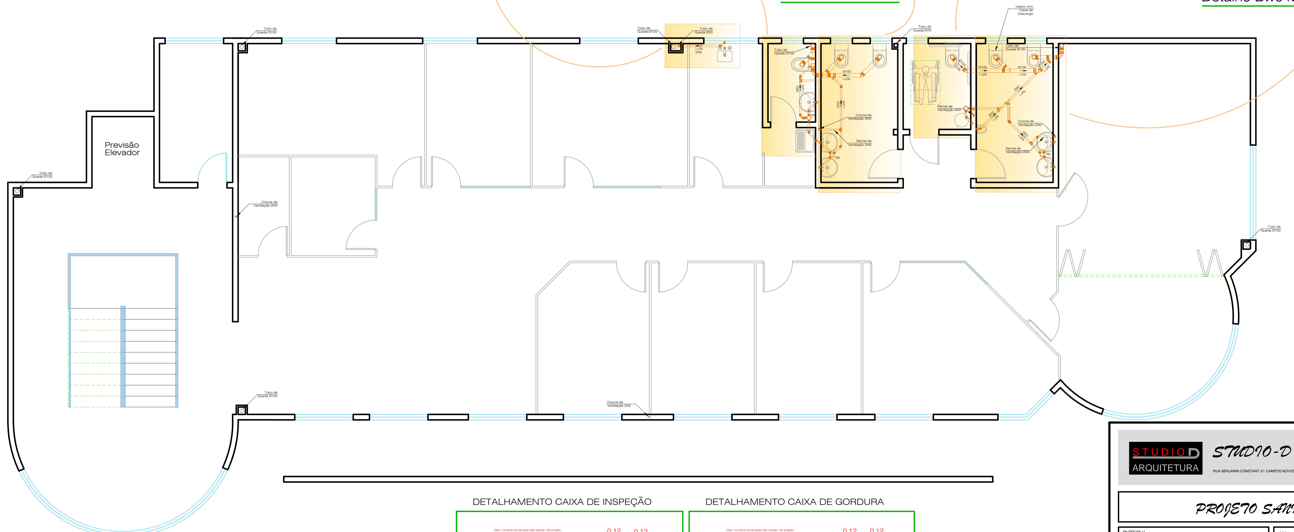
Planta de Instalação Sanitária - Pav. Superior Esc. 1:50
