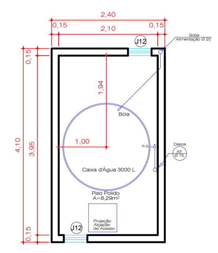
Planta de Reservatório Área = 9,84m 2 Esc. 1:50
