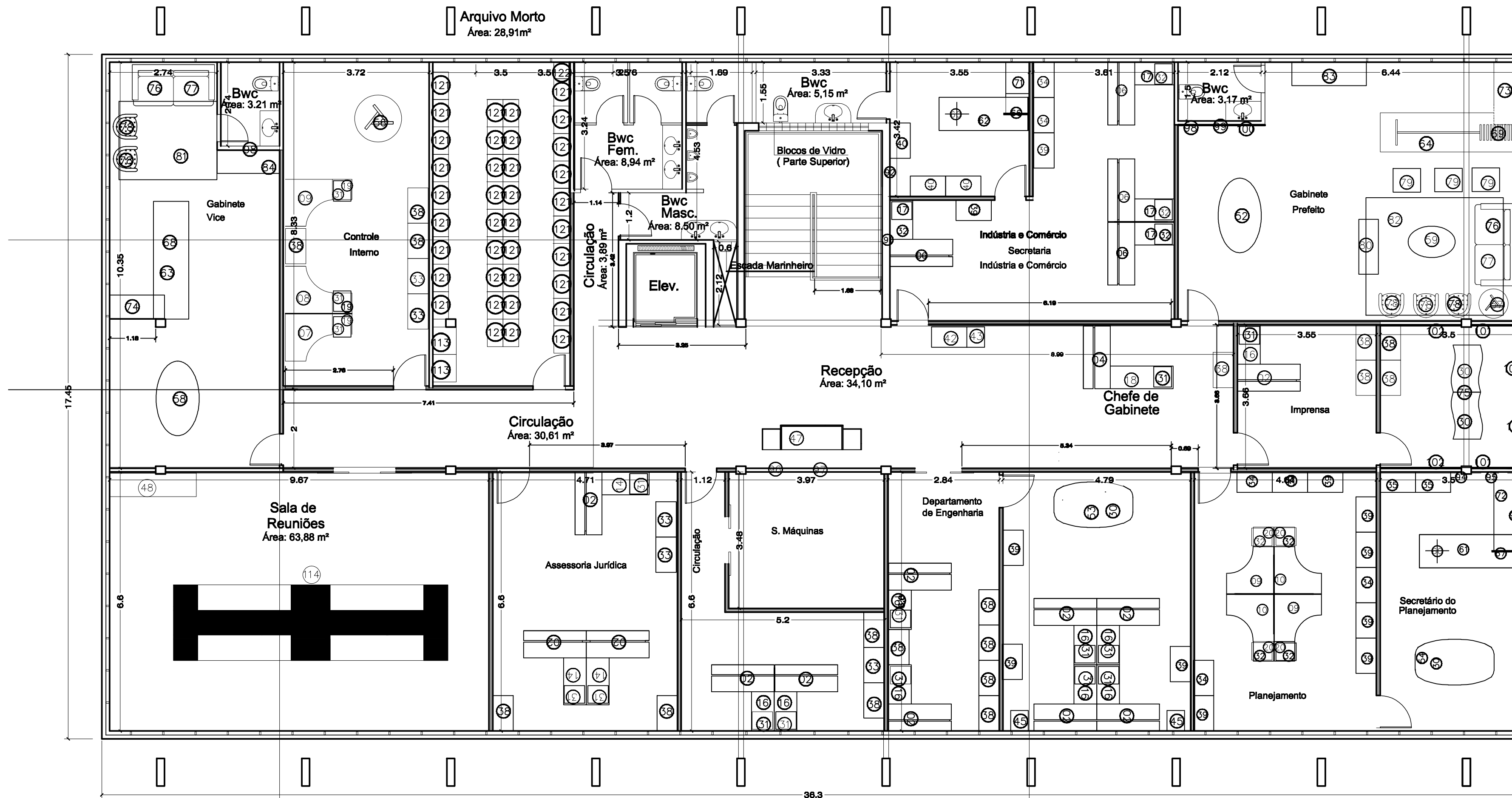
Planta Baixa Superior- Lay Out Mobiliário Esc: 1/75
