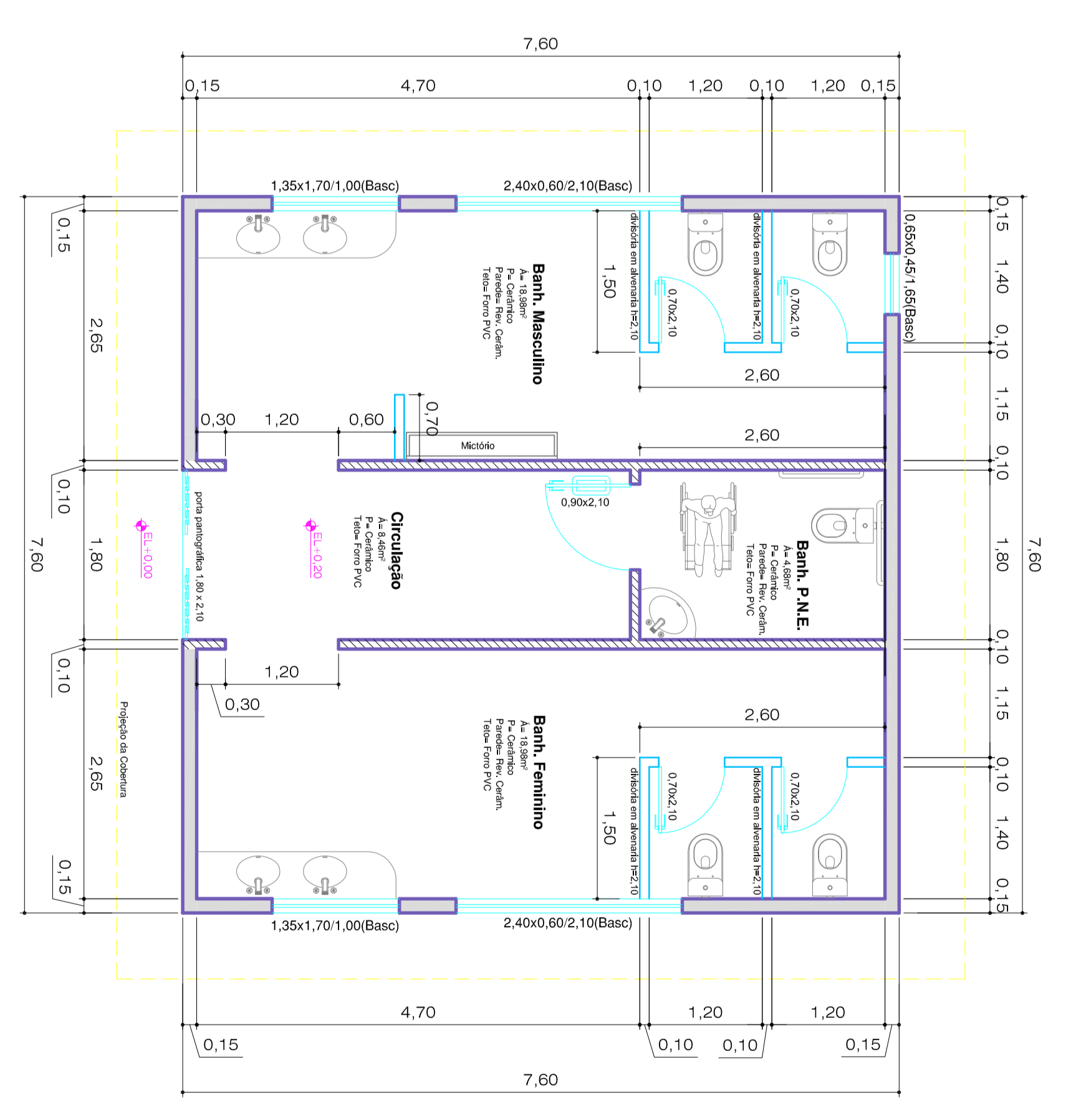
PLANTA BAIXA SANITÁRIOS (EDIFICAÇÃO A REFORMAR) Escala: 1:50
