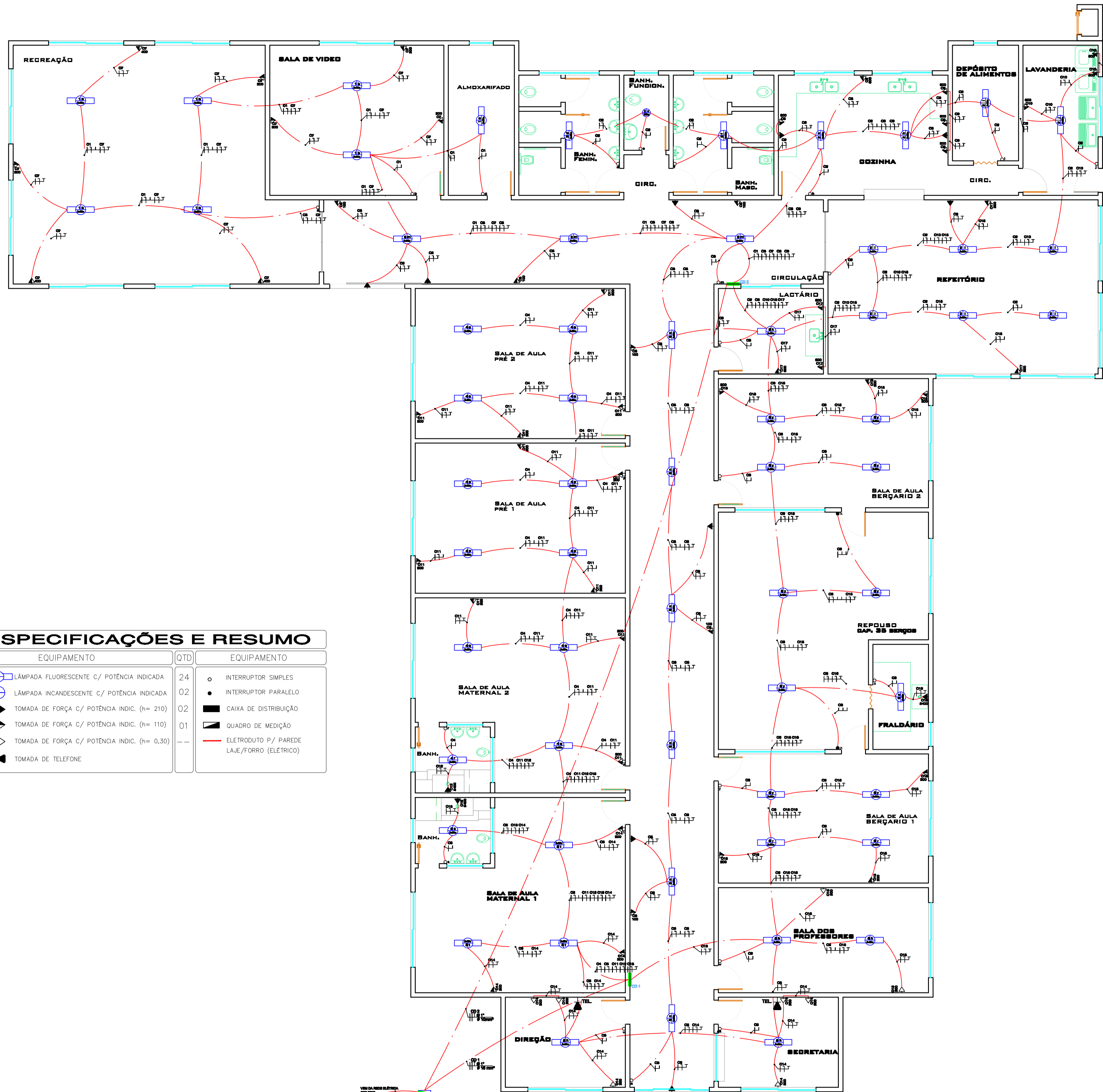
INSTALAÇÕES ELÉTRICAS ESCALA.....1:75
