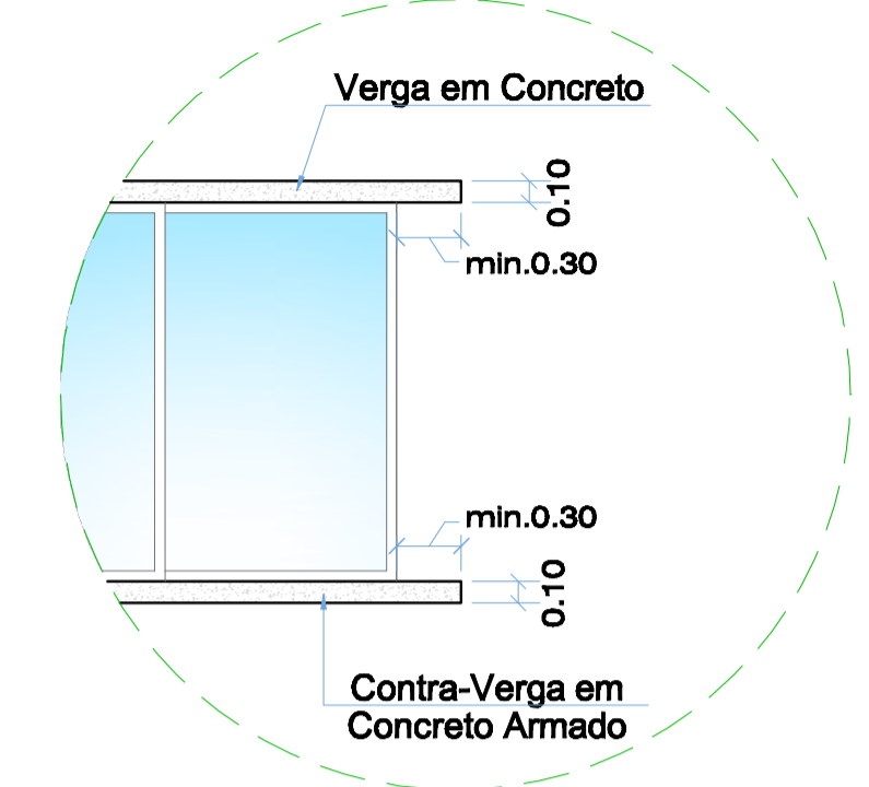
Det. 01 - Verga e Contra-Verga S/ESCALA
