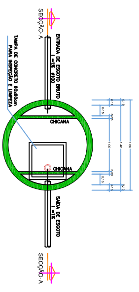
PLANTA BAIXA FOSSA SÉPTICA S/ ESCALA
