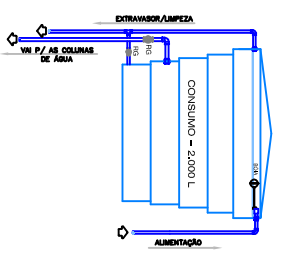
DETALHE RESERVATÓRIO S/ ESCALA
