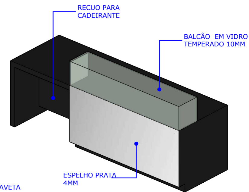
07 | PESPECTIVA 02 ESCALA.: 1/25
