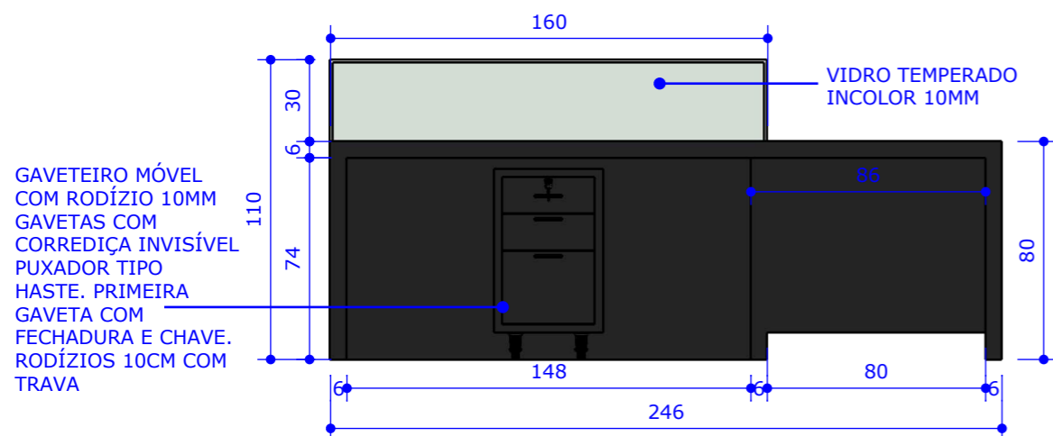
03 | VISTA POSTERIOR BALCÃO ESCALA.: 1/25
