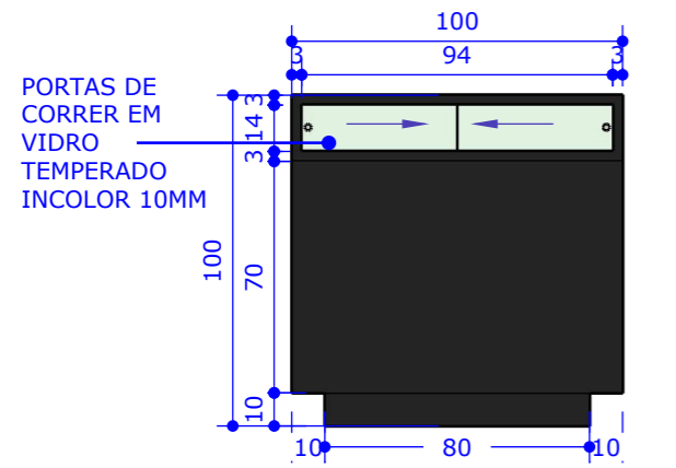
08 | VISTA POSTERIOR ESCALA.: 1/25
