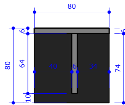
04 | CORTE 02 ESCALA.: 1/25
