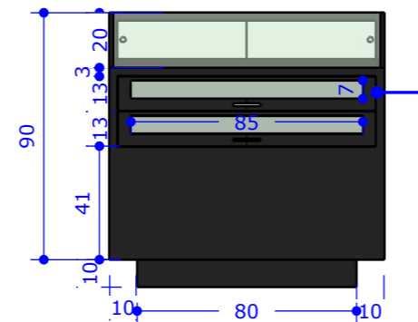
09 | VISTA FRONTAL ESCALA.: 1/25
