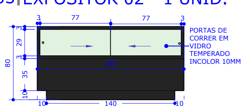
14 | VISTA POSTERIOR ESCALA.: 1/25
