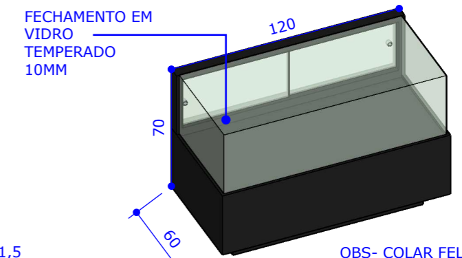
21 | PERSPECTIVA SEM ESCALA
