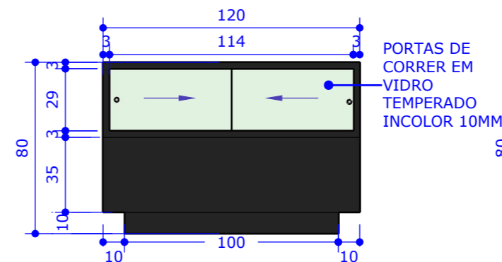
18 | VISTA POSTERIOR ESCALA.: 1/25
