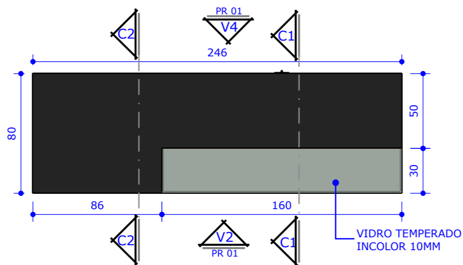
01 | VISTA FRONTAL BALCÃO ESCALA.: 1/25
