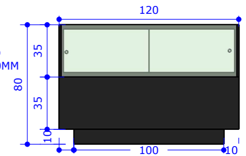
19 | VISTA FRONTAL ESCALA.: 1/25
