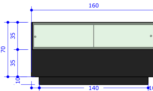
15 | VISTA FRONTAL ESCALA.: 1/25
