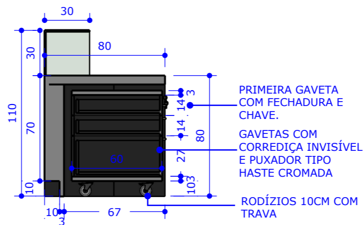
05 | CORTE 01 ESCALA.: 1/25
