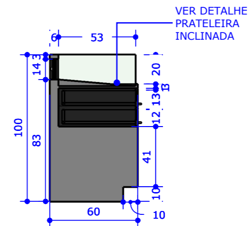
11 | CORTE 01 ESCALA.: 1/25
