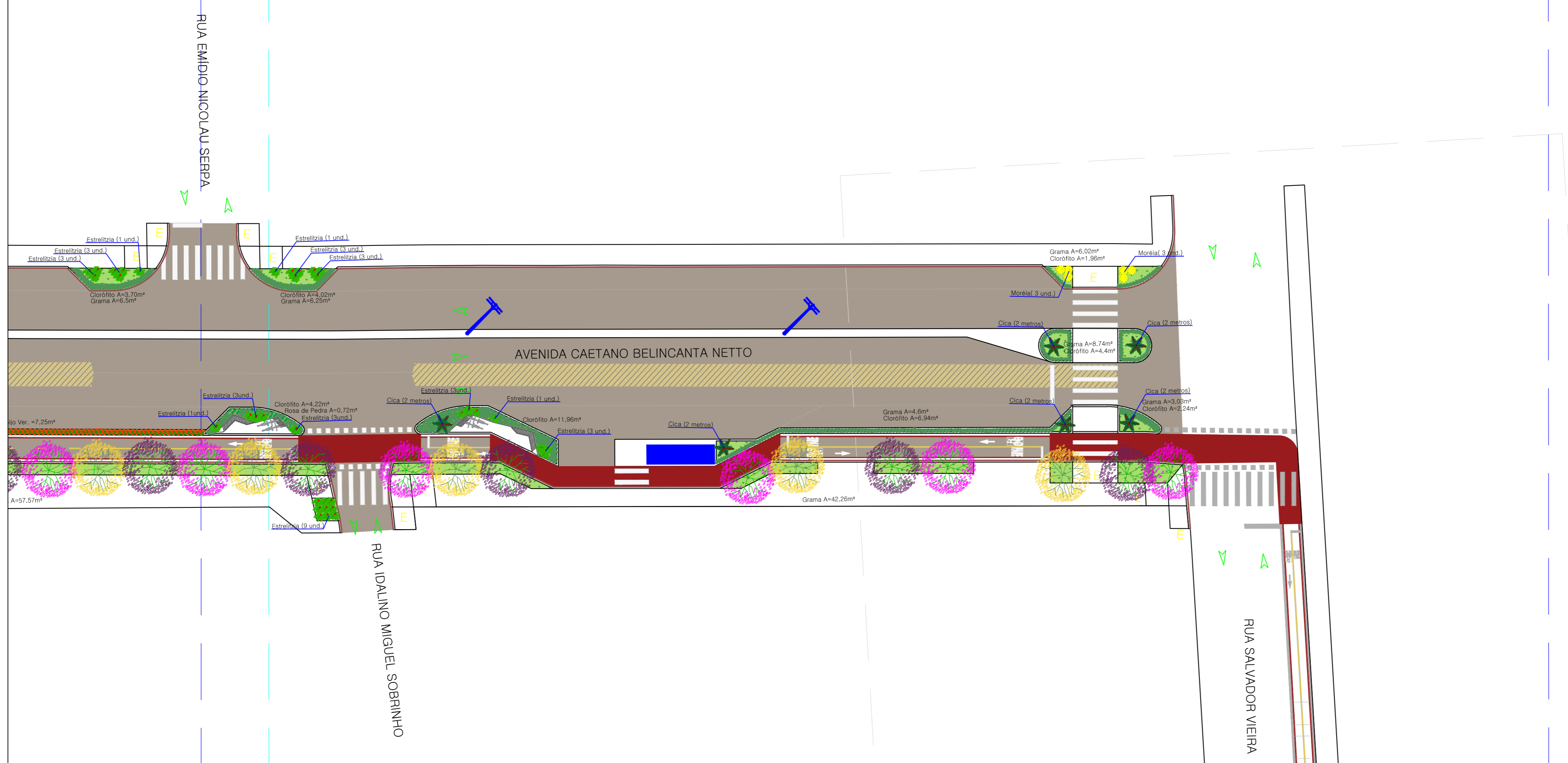
FOLHA 10/B ESCALA...: 1:250
