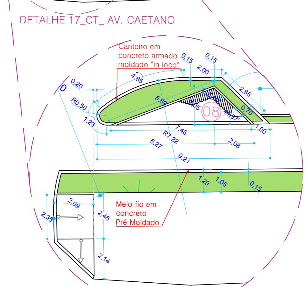
DETALHE 17 CANT. AV. CAETANO ESCALA...: 1:125
