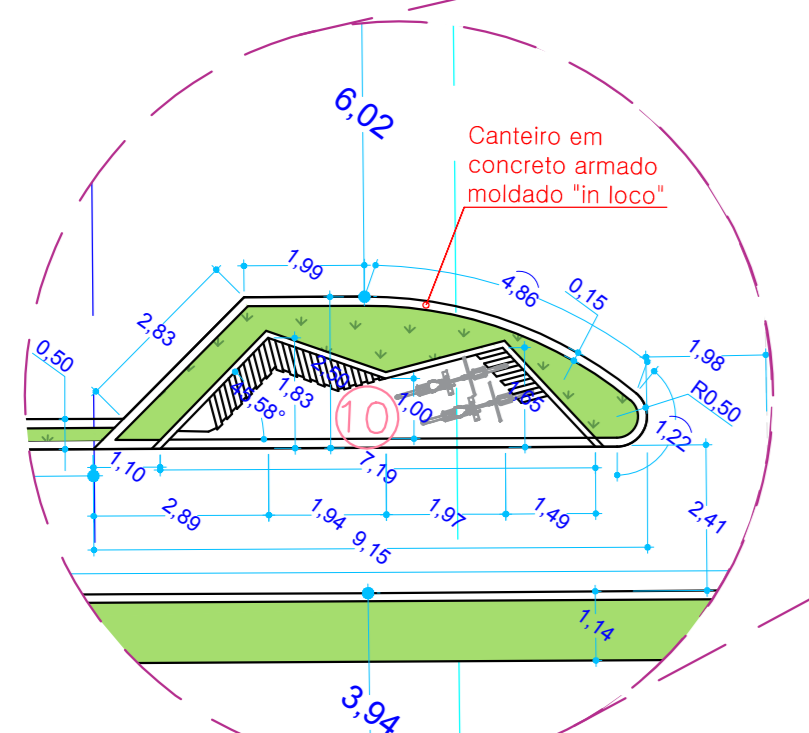
DETALHE 19 CANT. AV. CAETANO ESCALA...: 1:125
