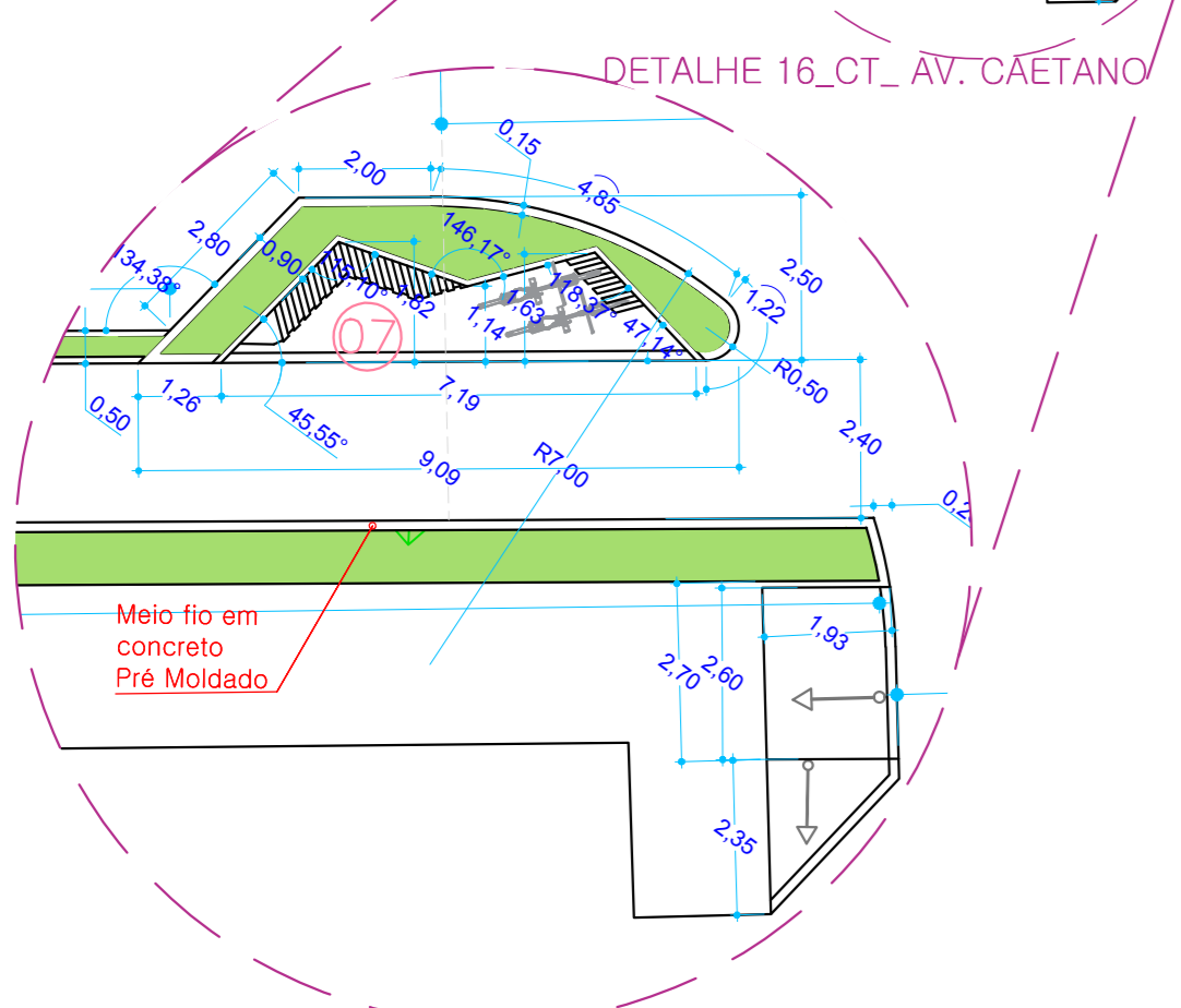
DETALHE 16 CANT. AV. CAETANO ESCALA...: 1:125
