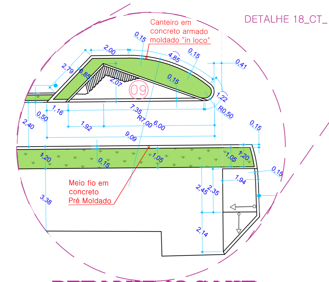
DETALHE 18 CANT. AV. CAETANO ESCALA...: 1:125
