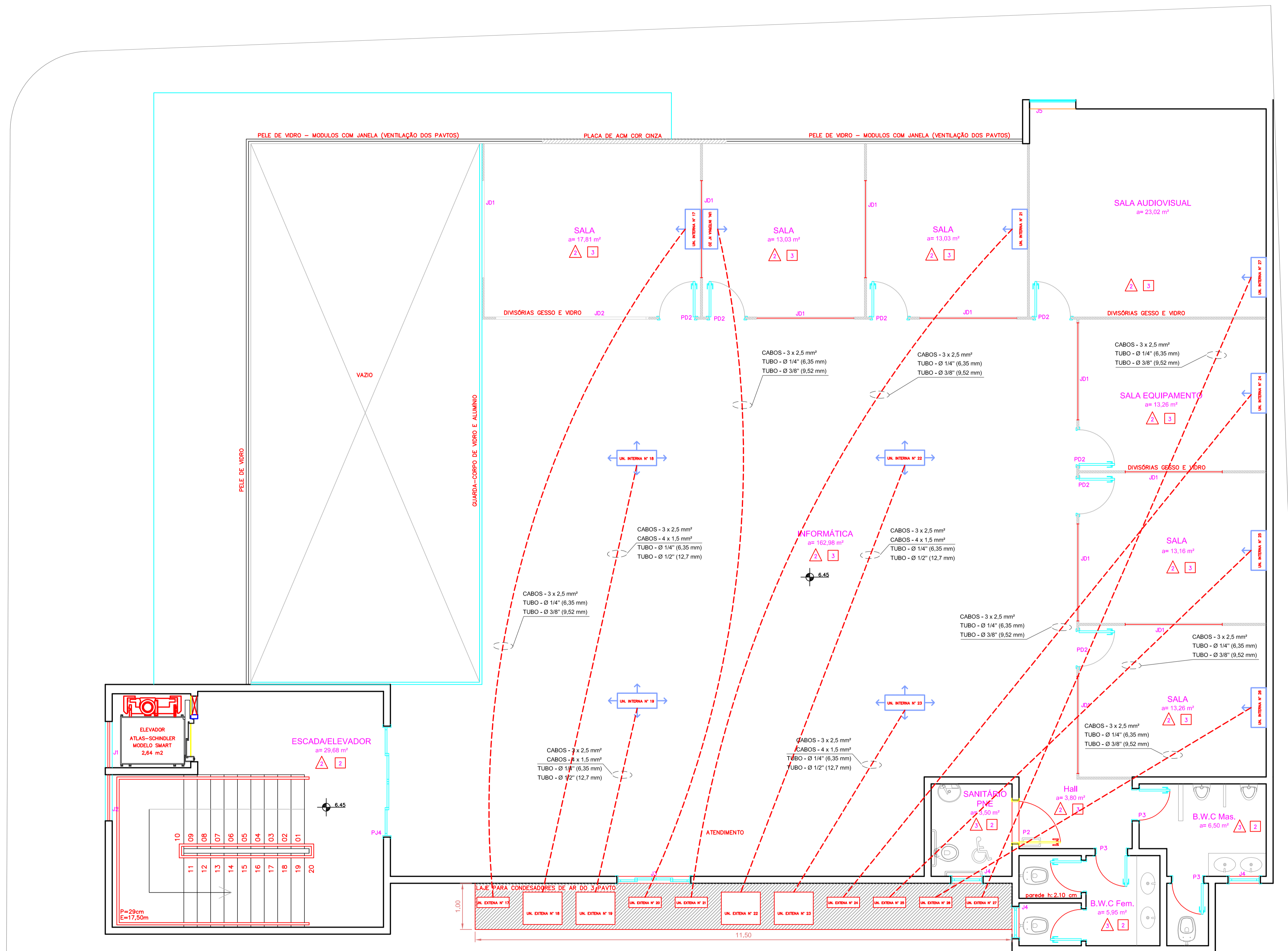
PLANTA BAIXA - 2º PAVIMENTO ÁREA = 331,50 m² Escala = 1/50
