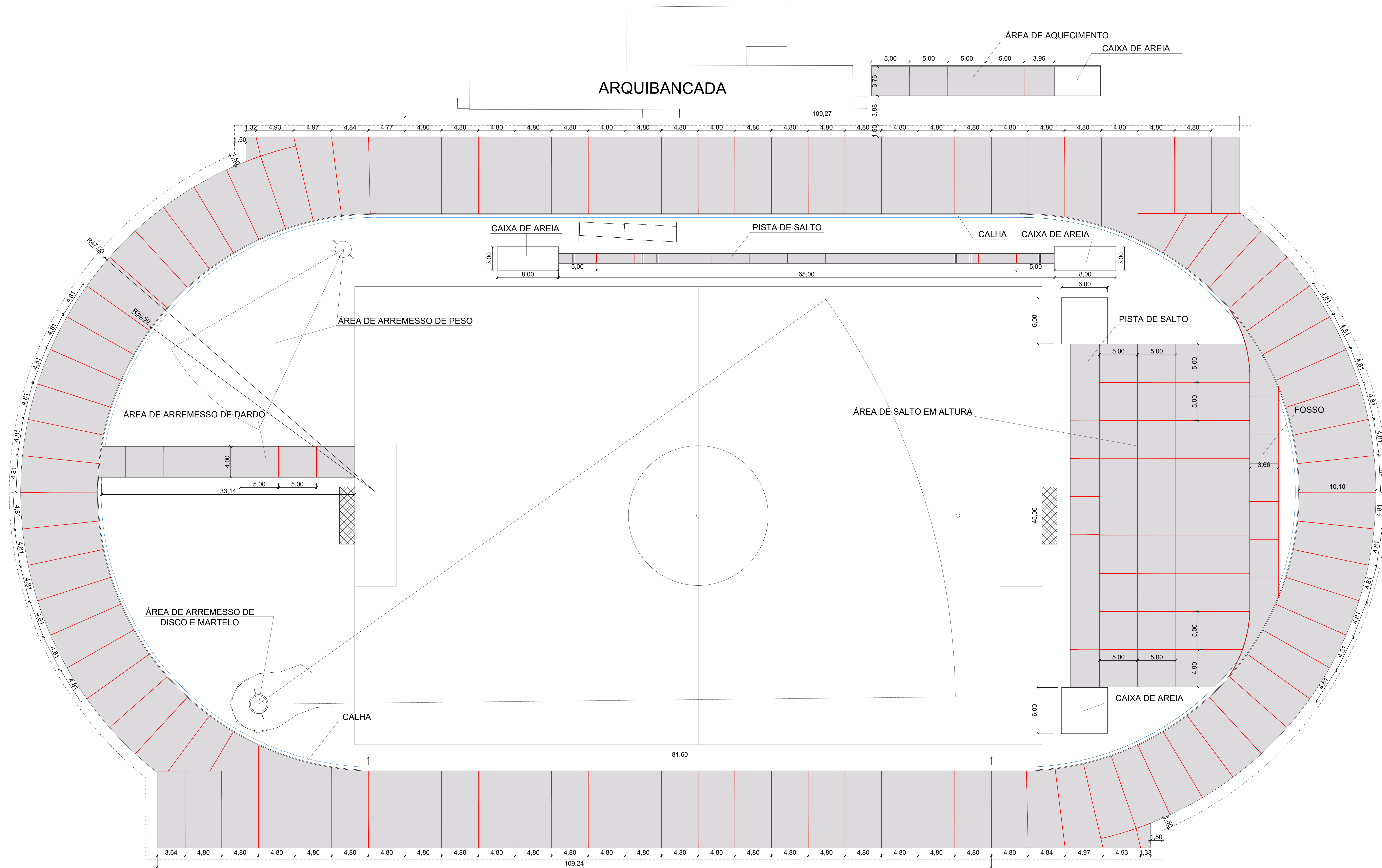
PISTA DE ATLETISMO ESCALA: 1/200
