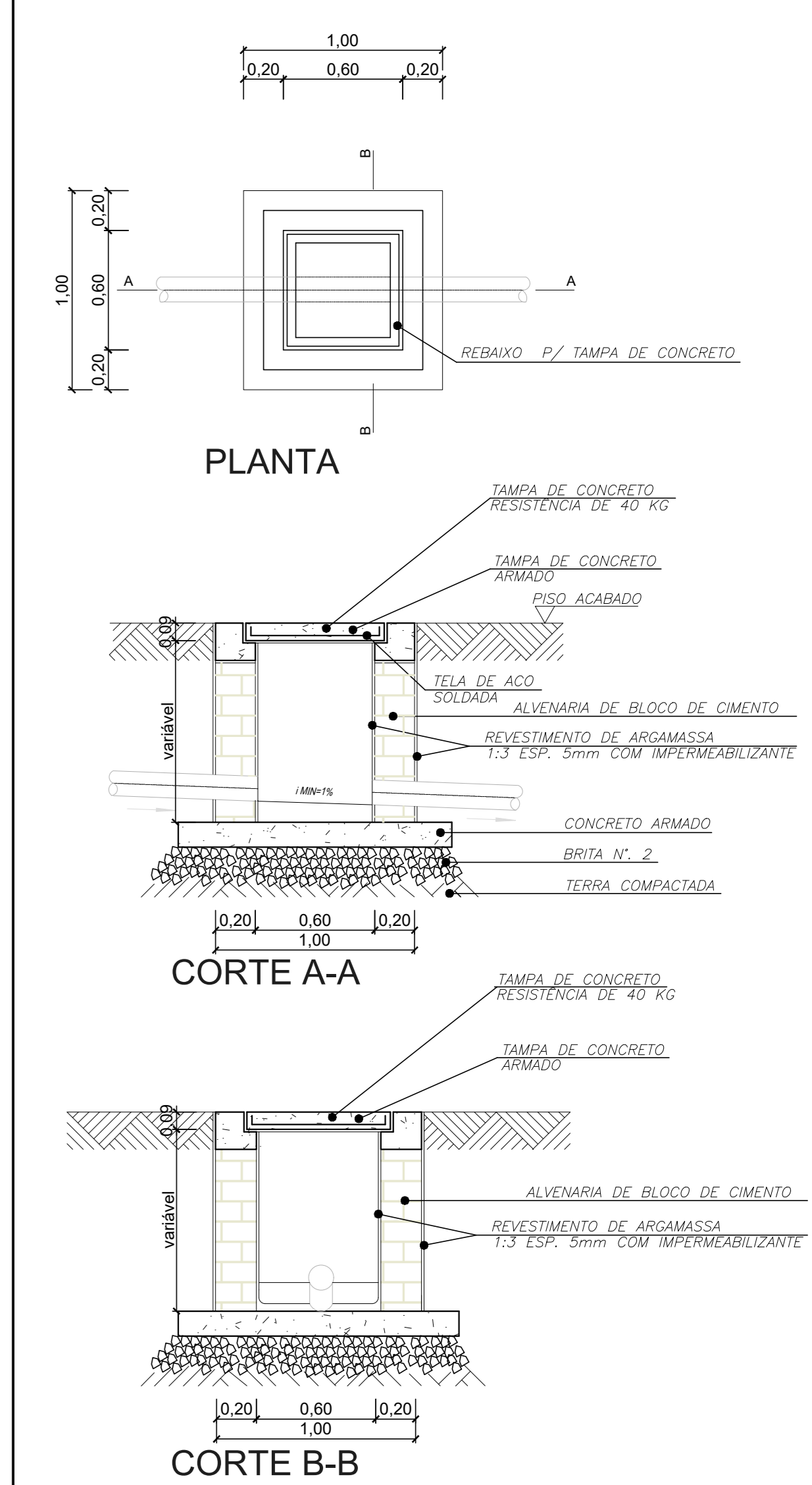
DETALHE CAIXA DE INSPEÇÃO DE ESGOTO ESC.: 1:25
