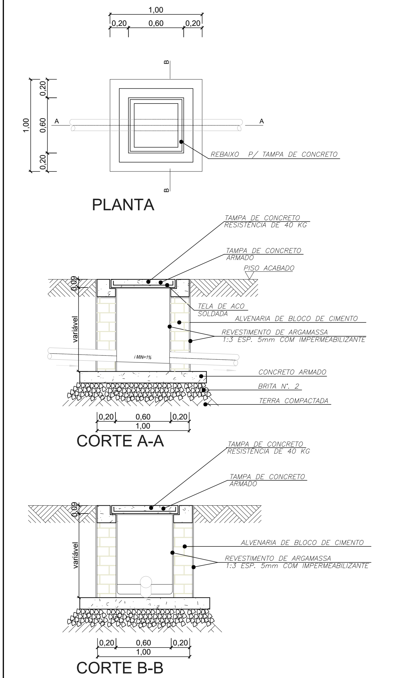
DETALHE CAIXA DE INSPEÇÃO DE ESGOTO ESC.: 1:25
