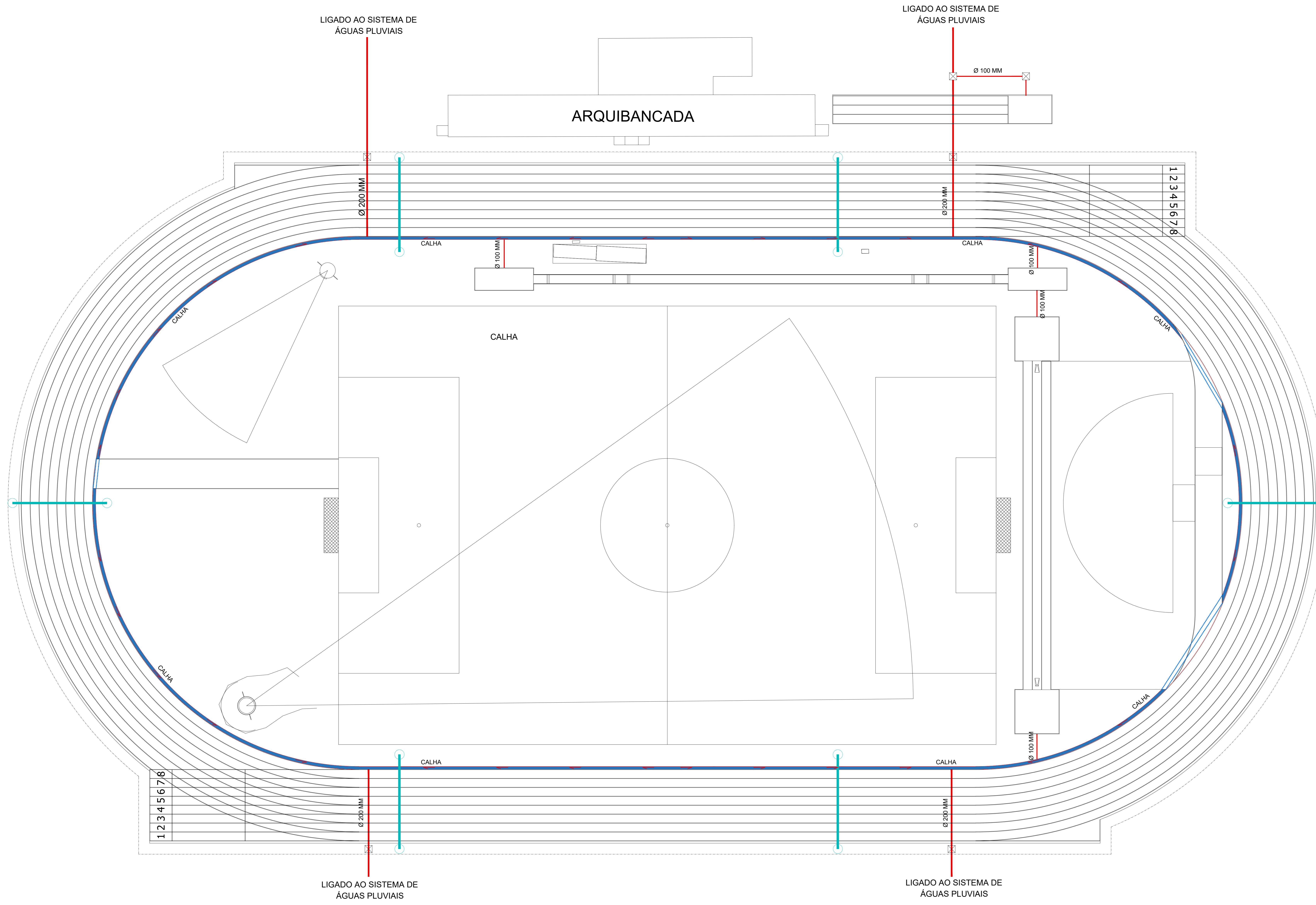
PISTA DE ATLETISMO ESCALA: 1/200
